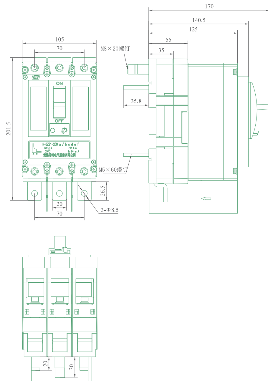
DZ931-250B/G 插入式安装电源侧板后负载侧板前接线(带电量附件或通信模块), 重量约4kg
