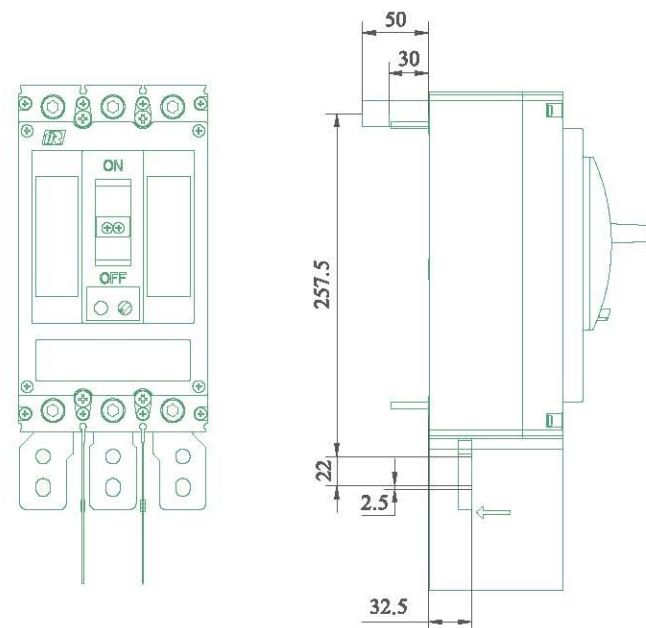
DZ931-630 固定式安装电源侧板后负载侧板前接线，重量约9.5kg
