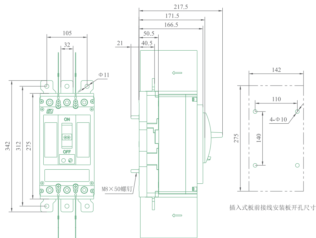
DZ931-400 插入式安装板前接线(可带电量附件)，重量约9.5kg
