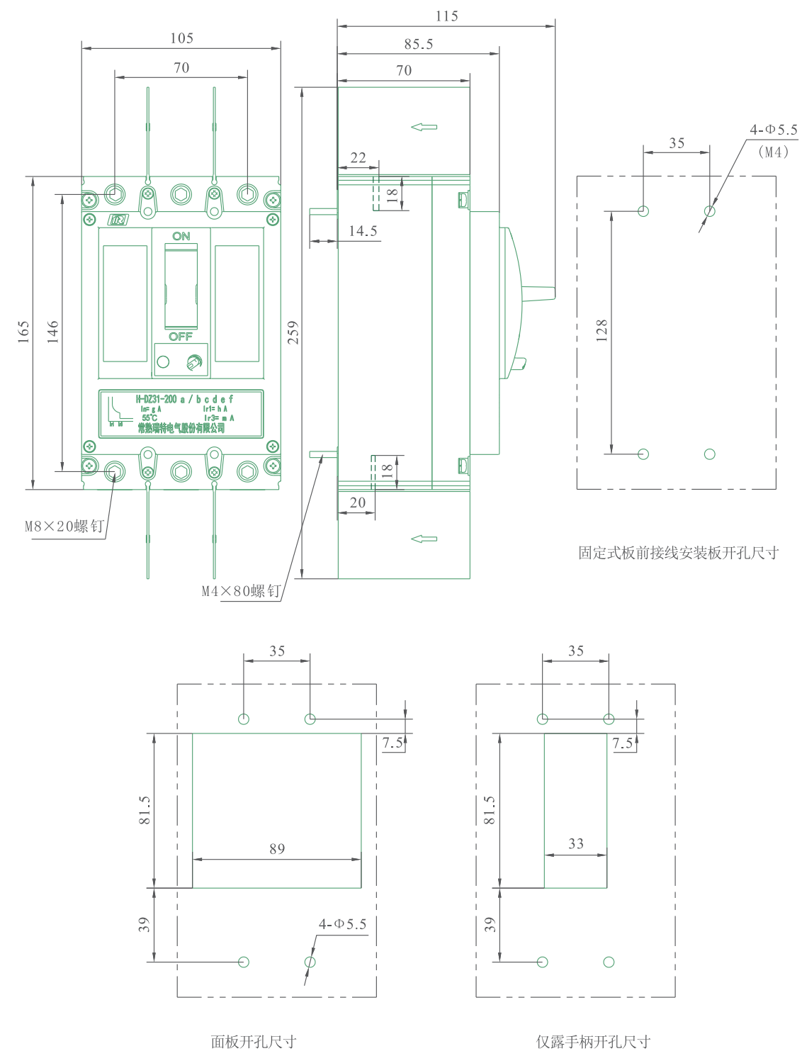
DZ931-250B/G 固定式安装板前接线, 重量约2.2kg
