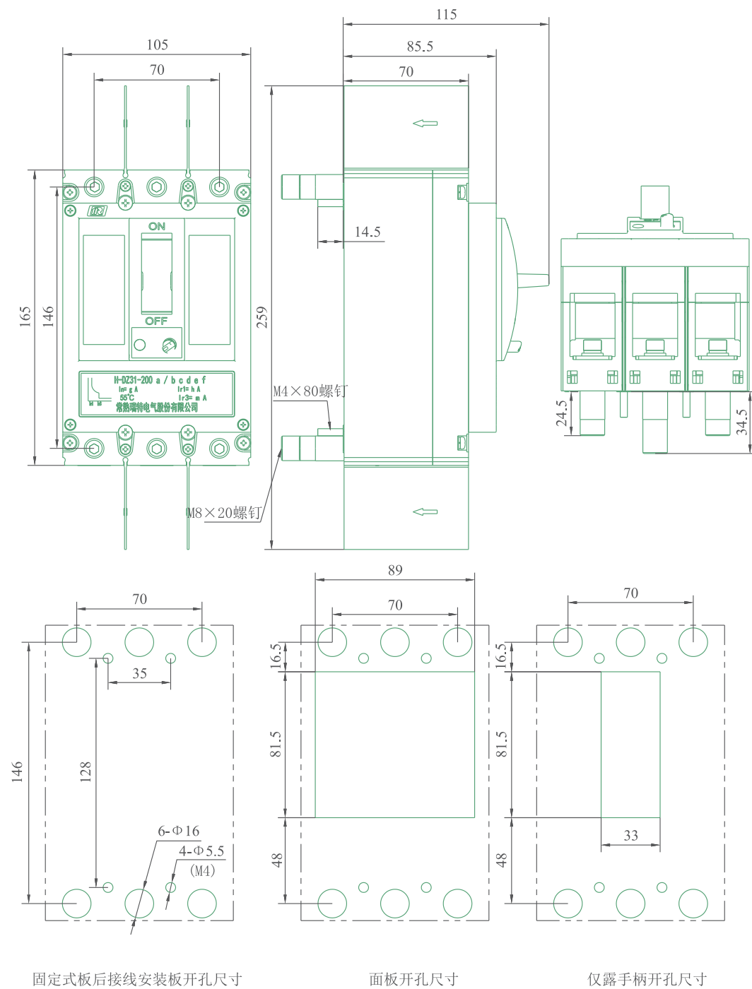
DZ931-250B/G 固定式安装板后接线，重量约2.5kg
