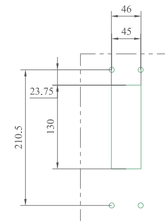
仅露手柄开孔尺寸
