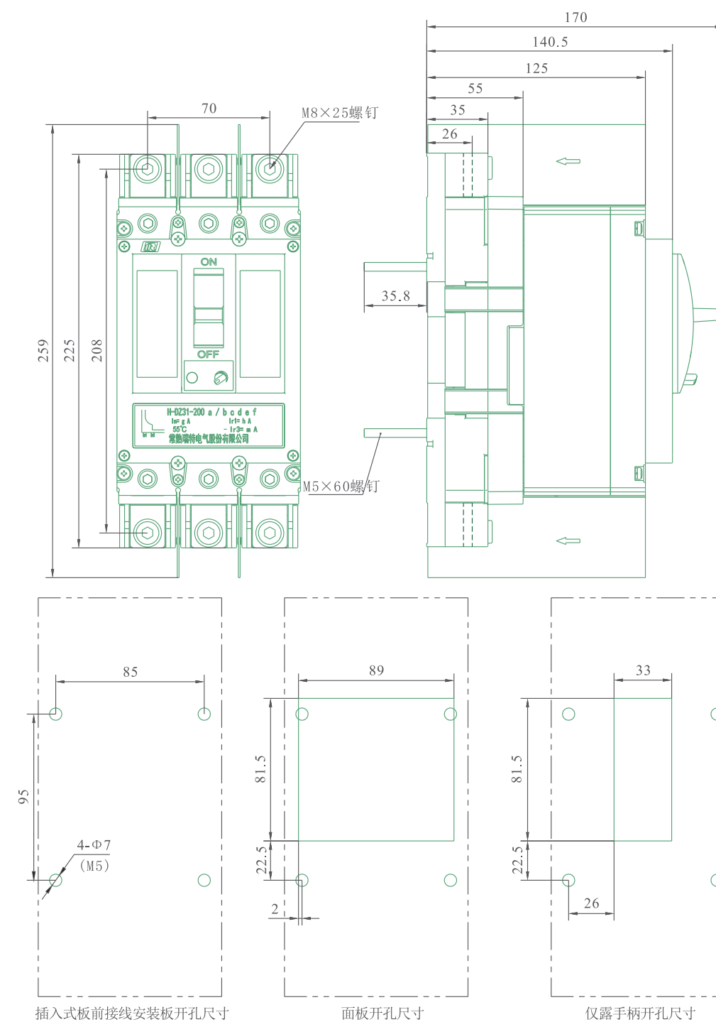
DZ931-250B/G 插入式安装板前接线(带电量附件或通信模块), 重量约4kg
