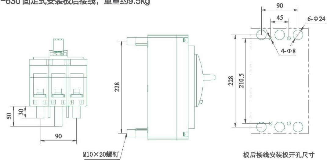
DZ931-630 固定式安装板后接线，重量约9.5kg
