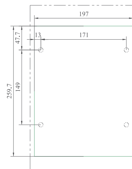
插入式面板开孔尺寸
