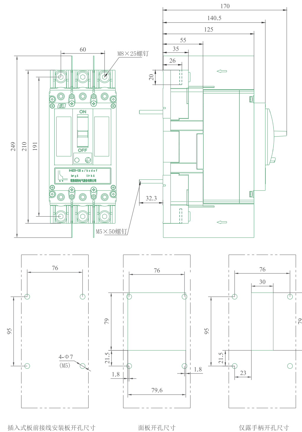
DZ931-125B/G 插入式安装板前接线(带电量附件或通信模块)(3P), 重量约3.4kg
