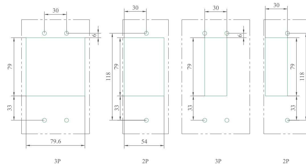
固定式面板开孔尺寸 (插入式板前开孔尺寸)
