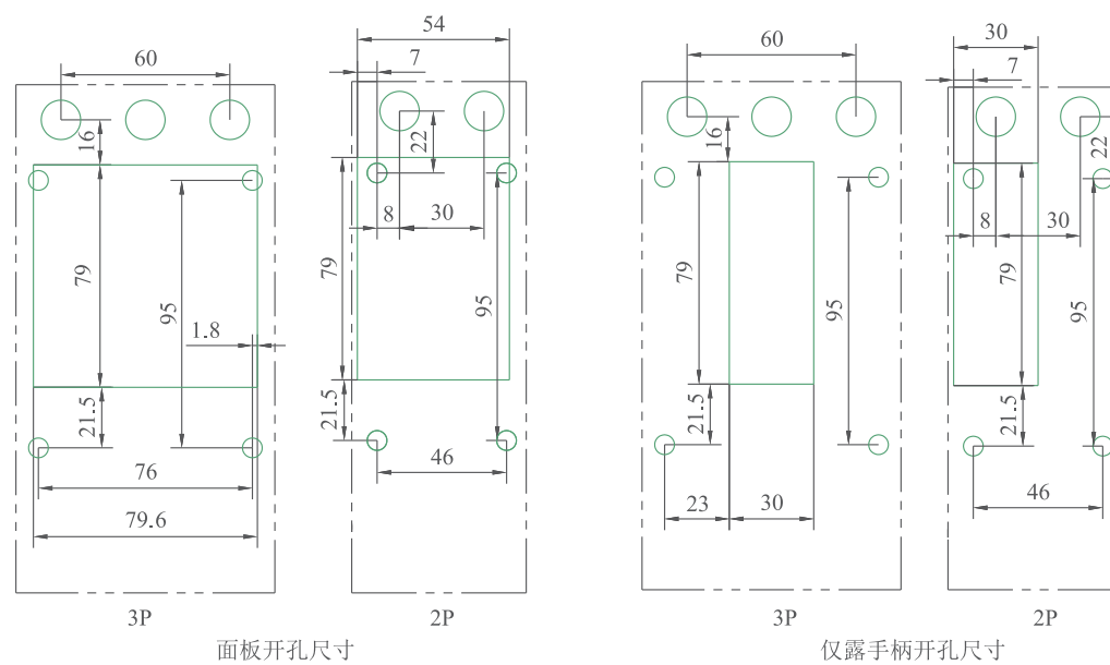
DZ931-125B/G插入式安装台电源侧板后负载侧板前面板开孔尺寸
