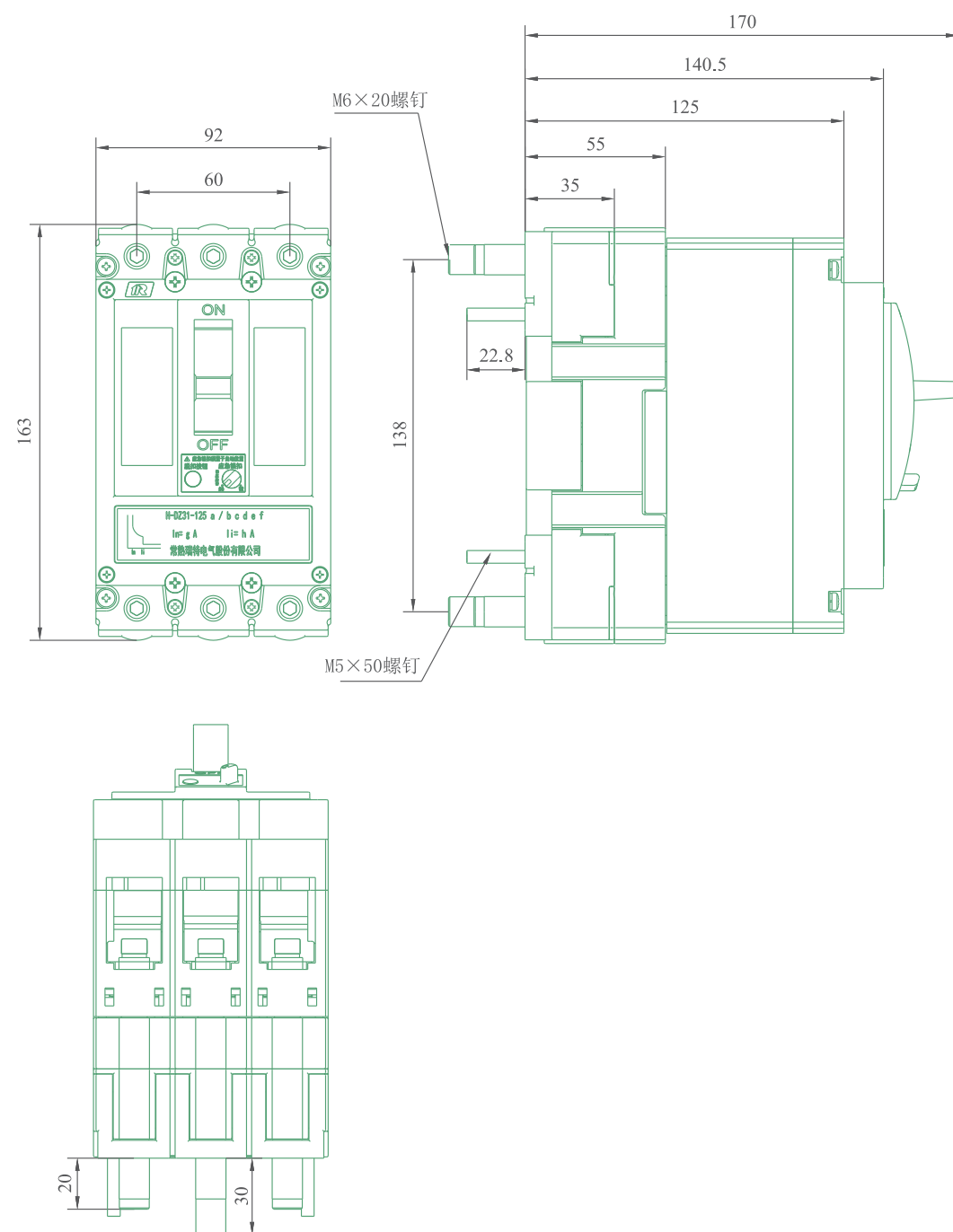
DZ931-125B/G 插入式安装板后接线(带电量附件或通信模块)(3P), 重量约3.4kg
