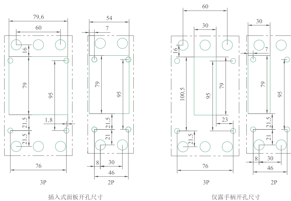
DZ931-125B/G插入式安装台电源侧板后负载侧板前面板开孔尺寸
