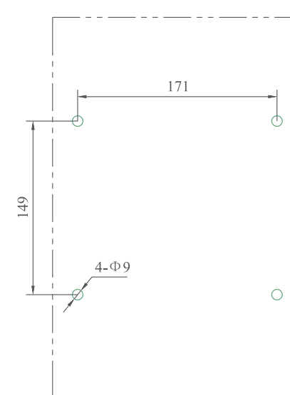
插入式板前接线安装板开孔尺寸
