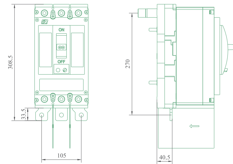
DZ931-400 插入式安装电源侧板前负载侧板后接线(可带电量附件)，重量约9.3kg
