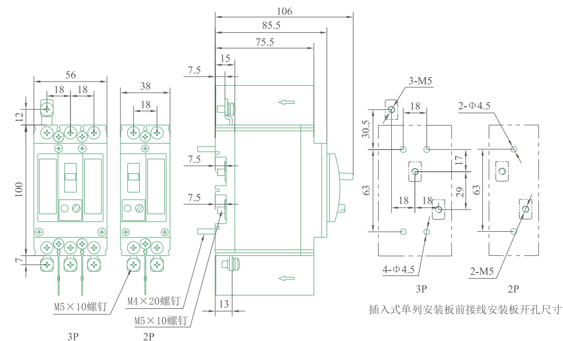
DZ931-50J 插入式单列安装板前接线，重量3P约0.8kg，2P约0.6kg
