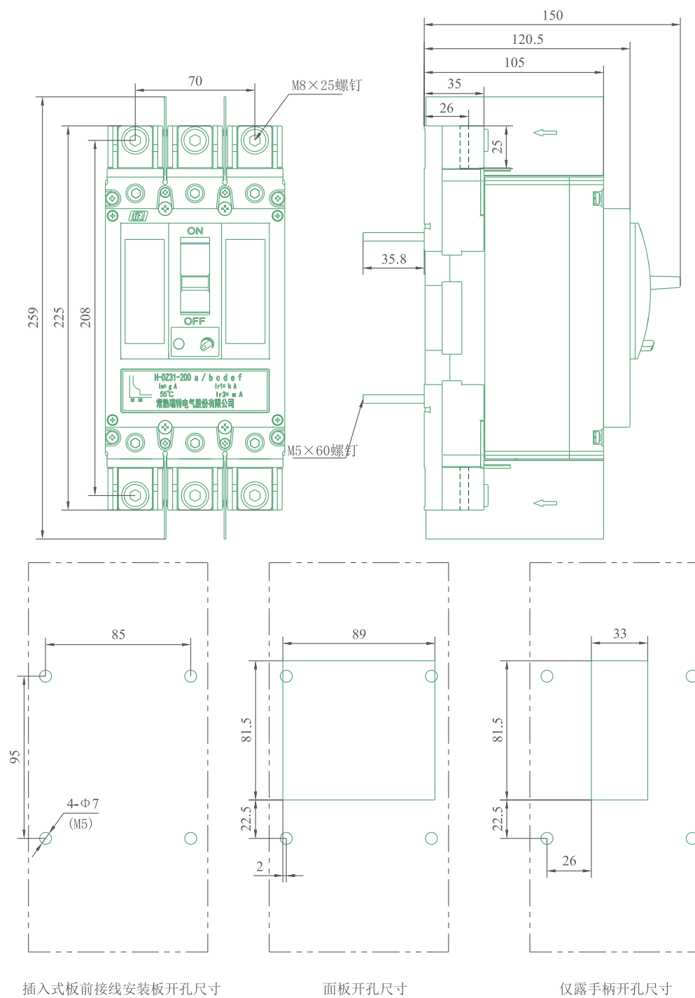
DZ931-250B/G 插入式安装板前接线，重量约3.5kg
