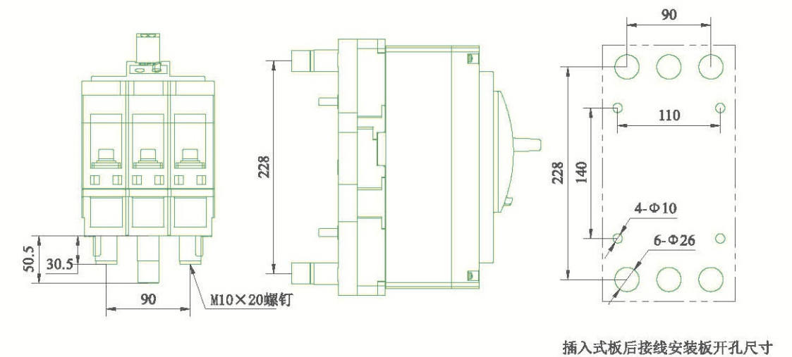
DZ931-630 插入式安装板后接线，重量约12kg
