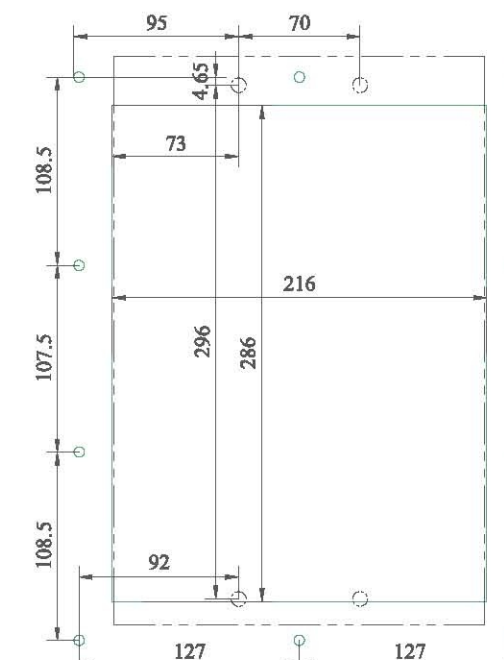
固定式带门框面板开孔尺寸
