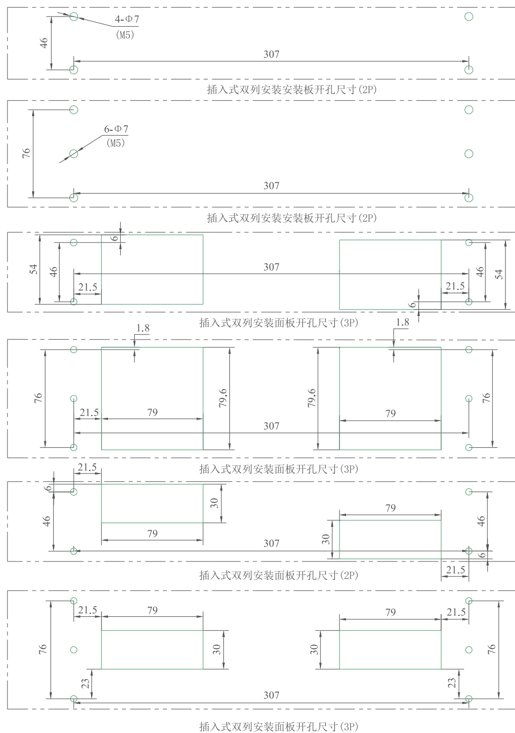
DZ931-125B/G 插入式双列安装板前接线面板开孔尺寸
