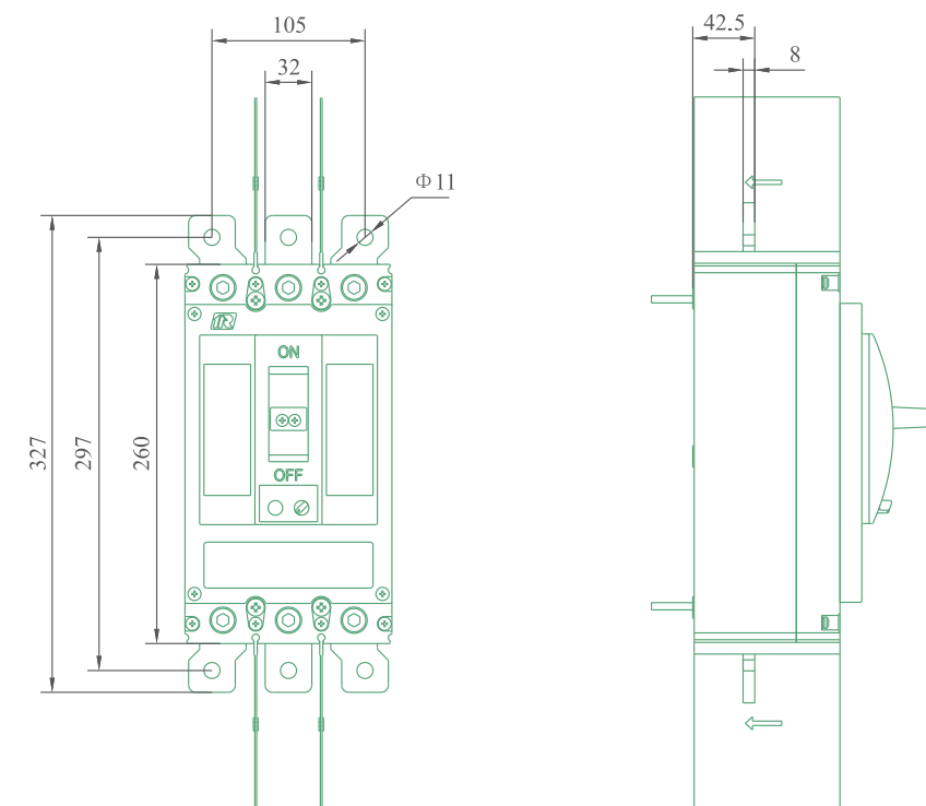
DZ931-400 固定式安装板前接线加转接排，重量约6.5kg
