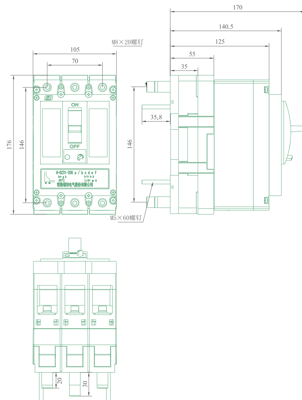
DZ931-250B/G 插入式安装板后接线(带电量附件或通信模块), 重量约4kg
