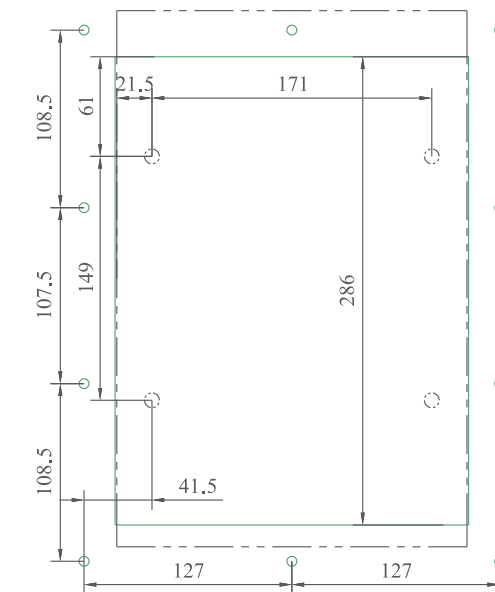
插入式带门框面板开孔尺寸
