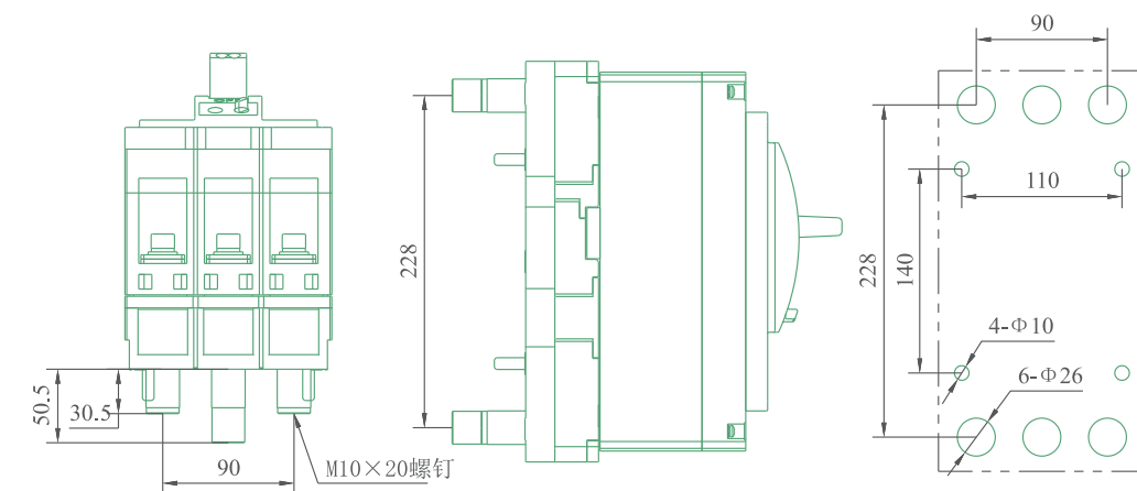
插入式板后接线安装板开孔尺寸
