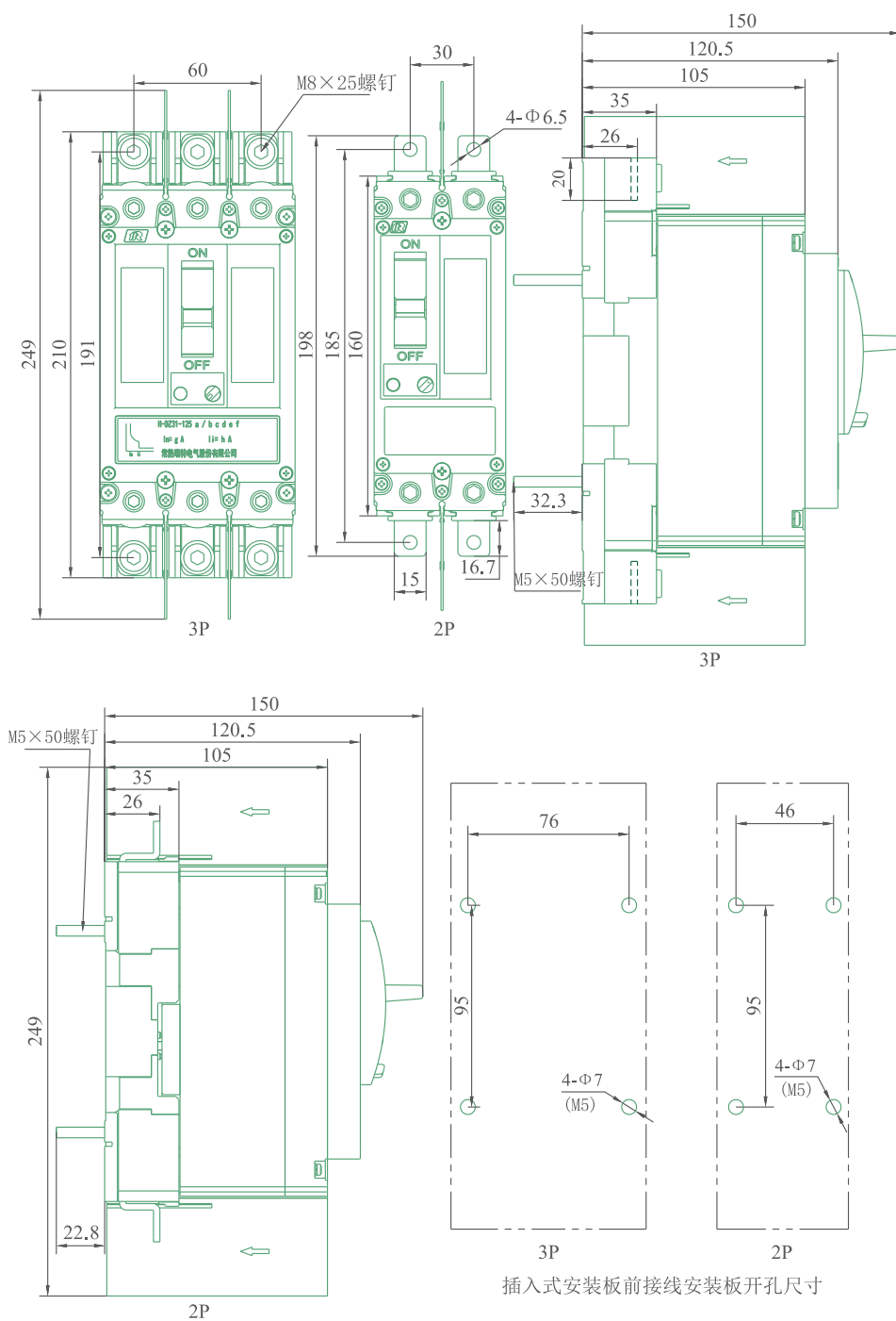
DZ931-125B/G 插入式安装板前接线，重量3P约3kg，2P约2kg
