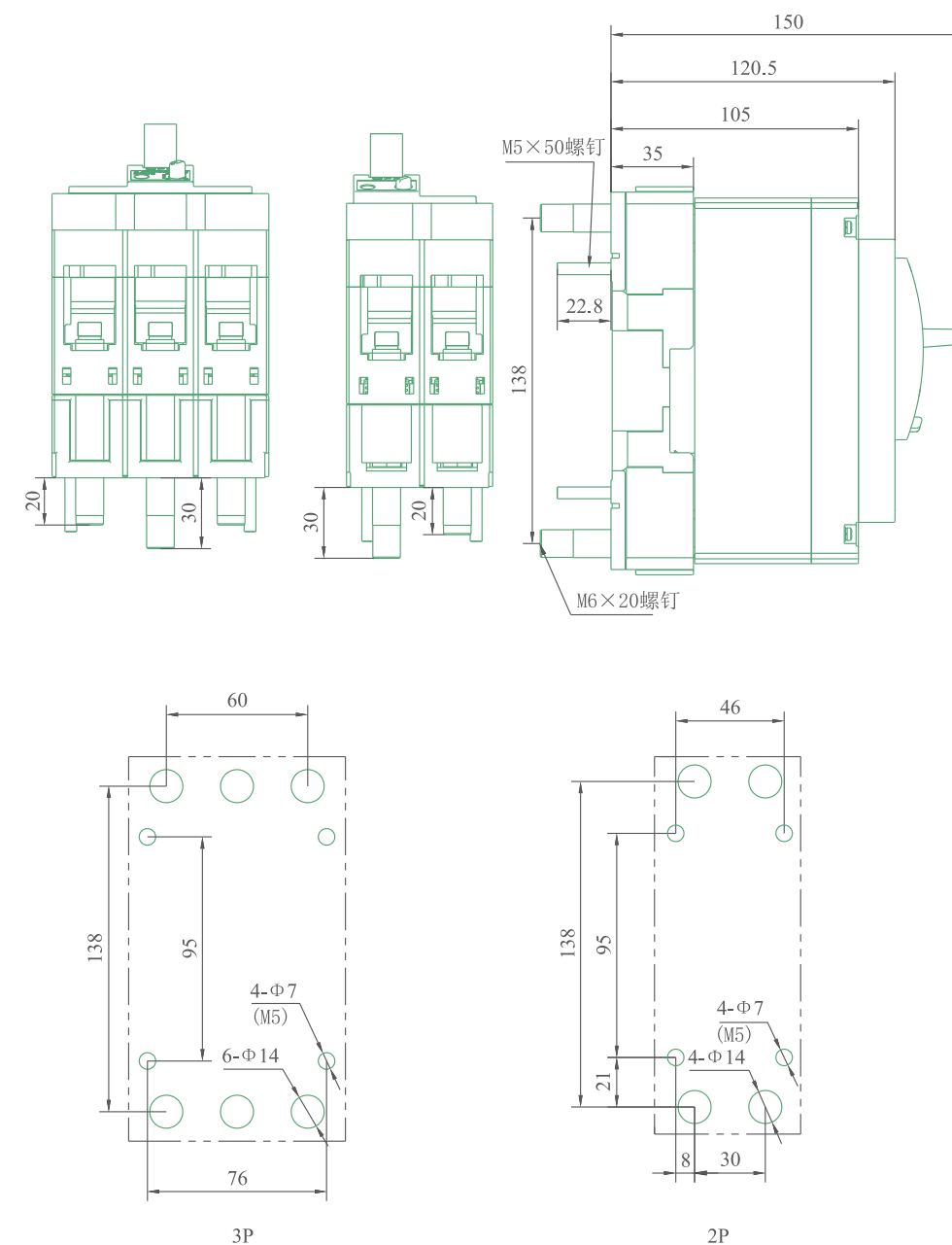
插入式安装板后接线安装板开孔尺寸
