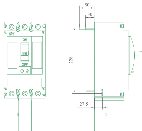
DZ931-400 固定式安装电源侧板后负载侧板前接线，重量约6.3kg
