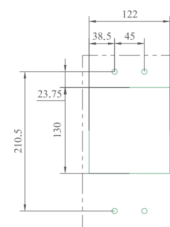
面板开孔尺寸
