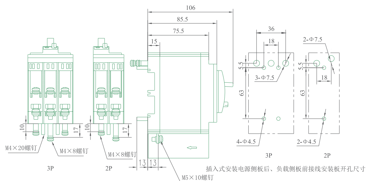
DZ931-50J 插入式安装电源侧板后负载侧板前接线，重量3P约0.8kg，2P约0.6kg
