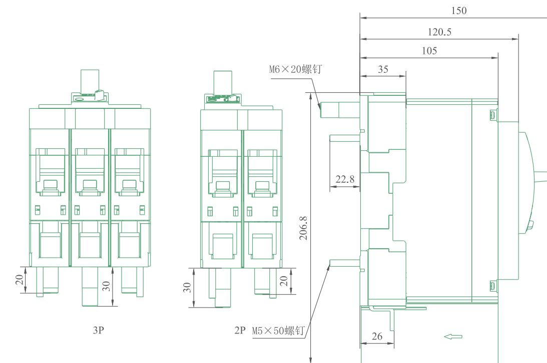
DZ931-125B/G 插入式安装电源侧板后负载侧板前接线，重量3P约3kg，2P约2kg
