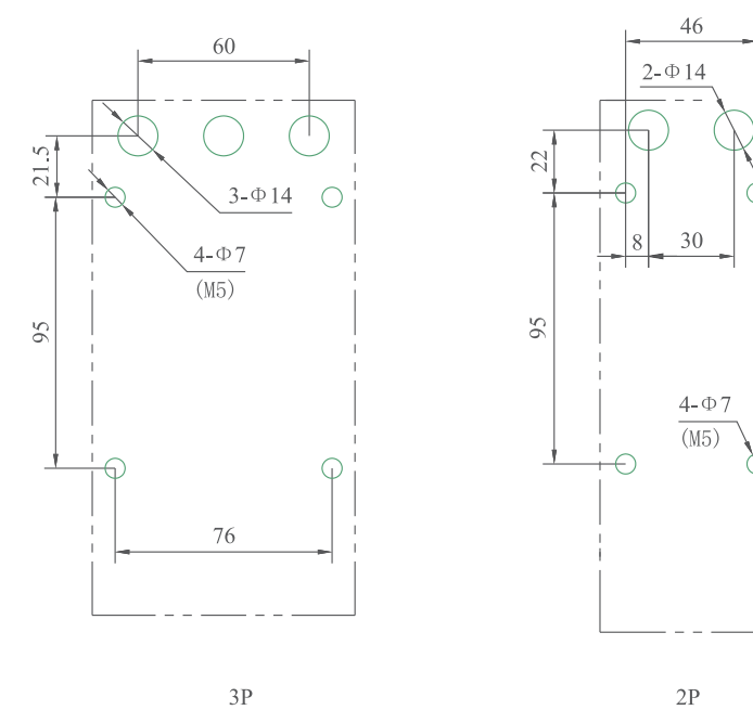
插入式安装台电源侧板后负载侧板前安装开孔尺寸
