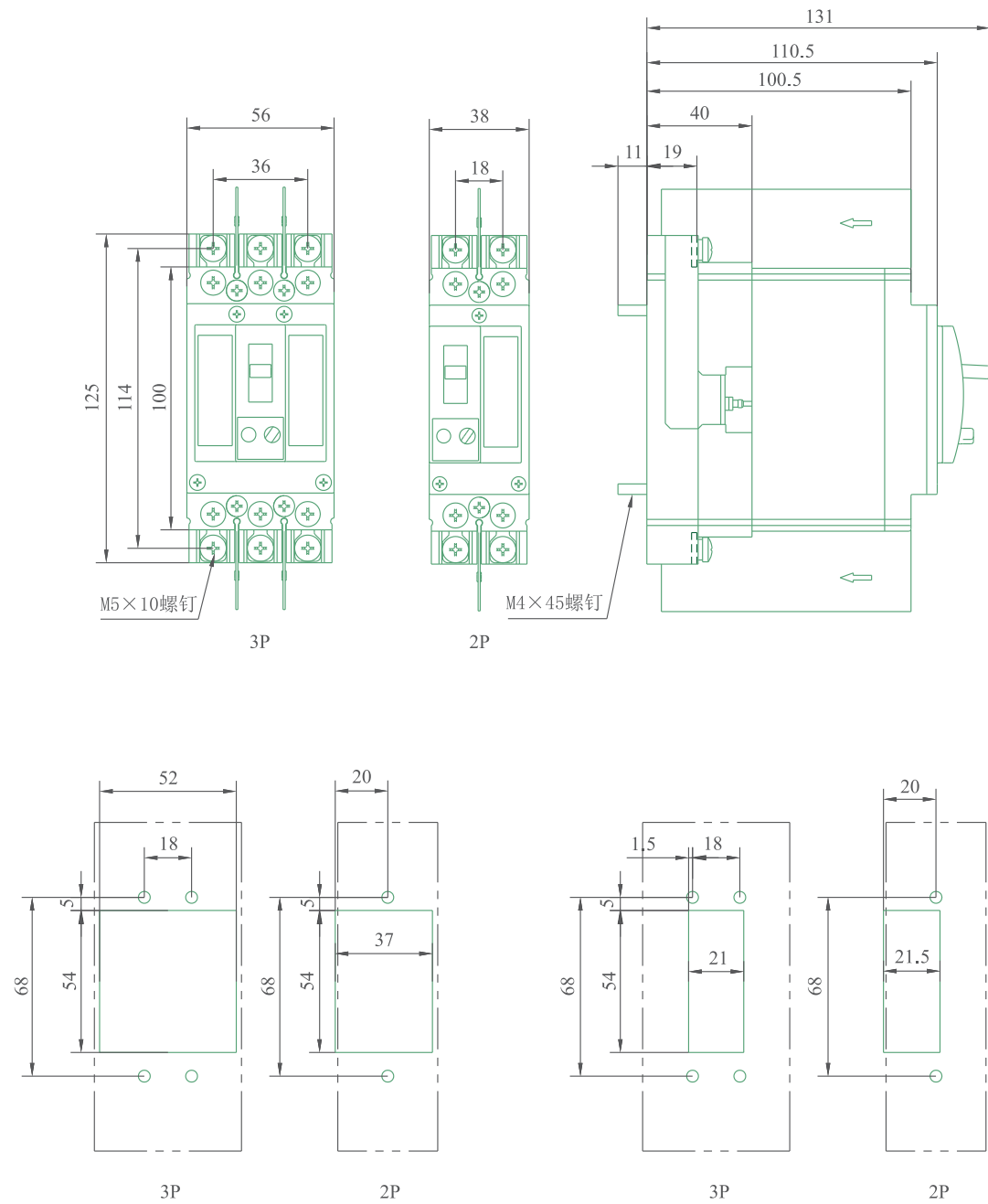
DZ931-50J 插入式安装板前接线(带电量附件), 重量3P约1kg, 2P约0.8kg
