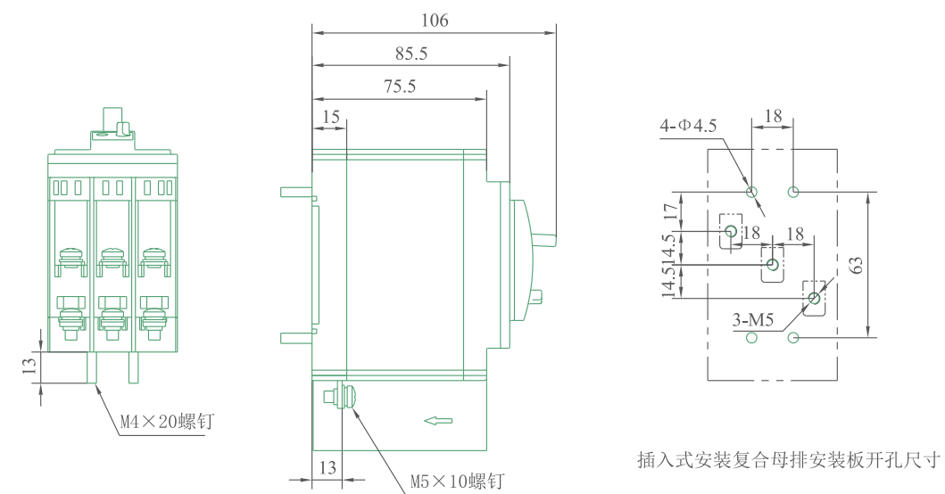
DZ931-50J 插入式安装复合母排接线，重量3P约0.8kg
