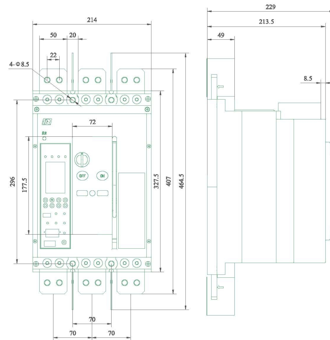
DZ931-1250 固定式安装板前接线(内置电操)，重量约23kg
