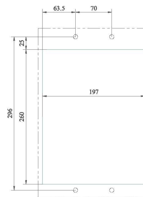
固定式面板开孔尺寸
