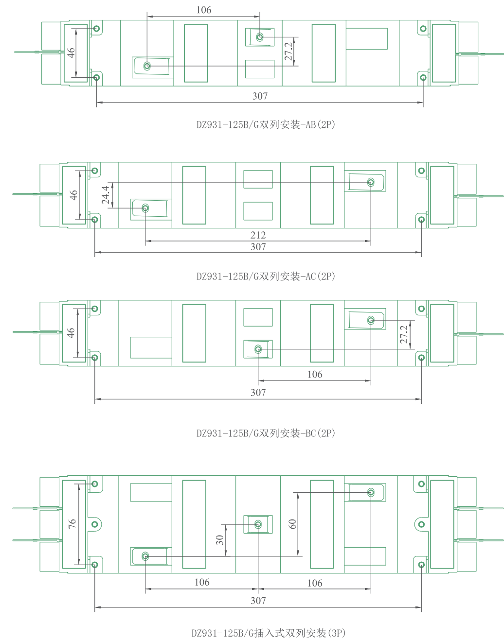
DZ931-125B/G 插入式双列安装母线位置
