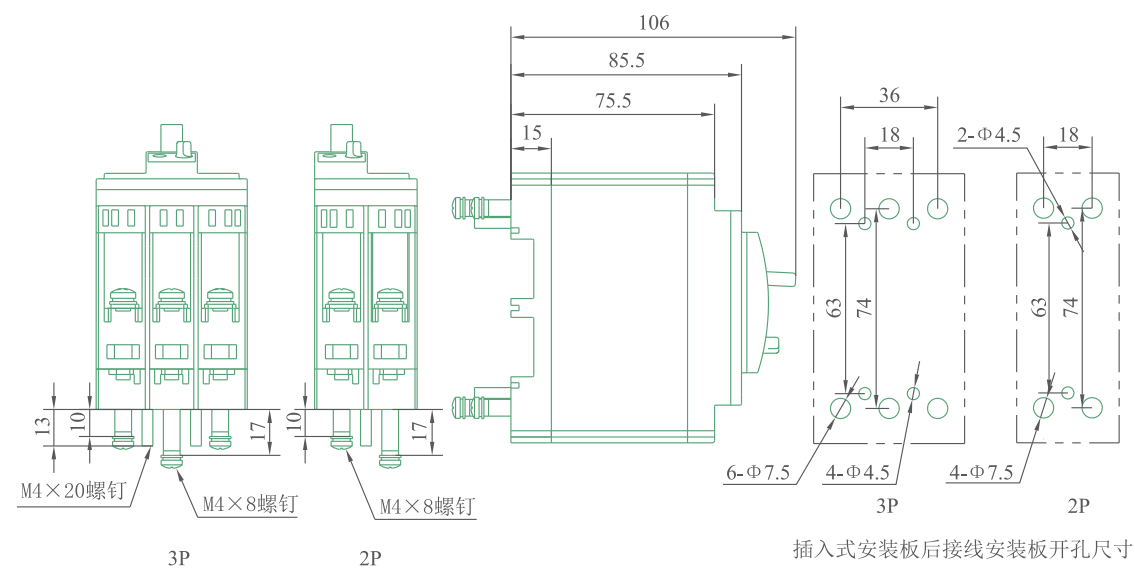
DZ931-50J 插入式安装板后接线，重量3P约0.8kg，2P约0.6kg
