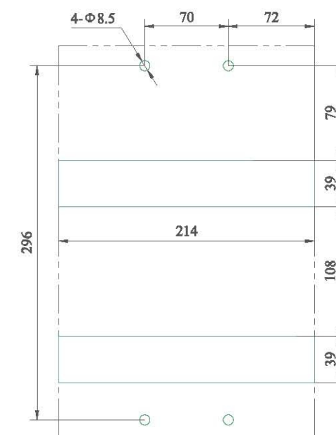
固定式板后接线安装板开孔尺寸
