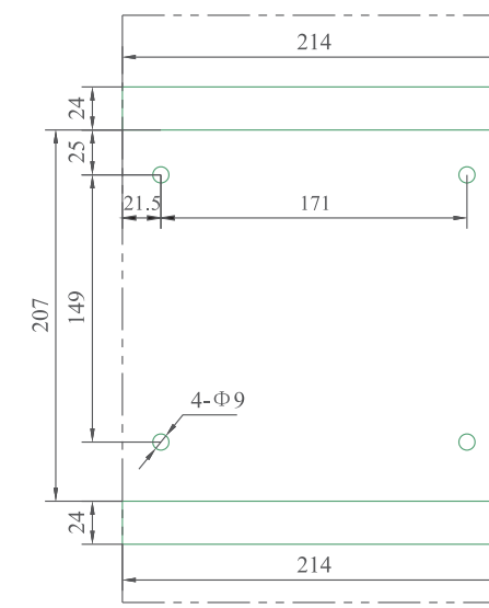
插入式板后接线安装板开孔尺寸
