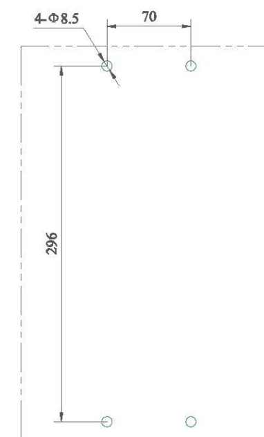
固定式板前接线安装板开孔尺寸
