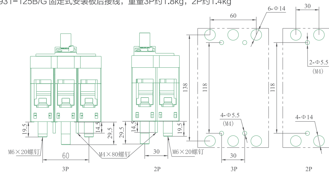
固定式板后接线安装板开孔尺寸
