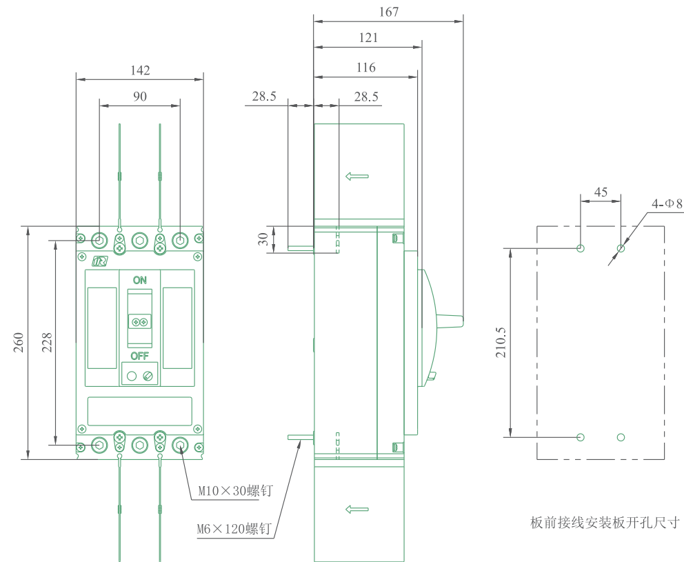
DZ931-400 固定式安装板前接线，重量约6kg
