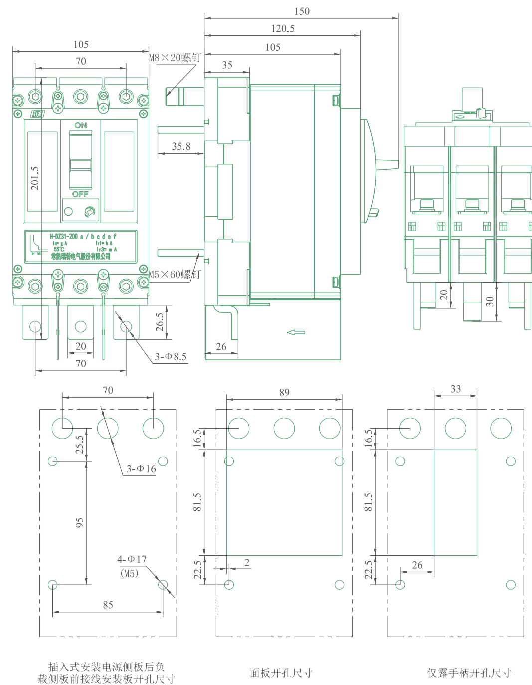
DZ931-250B/G 插入式安装电源侧板后负载侧板前接线，重量约3.5kg
