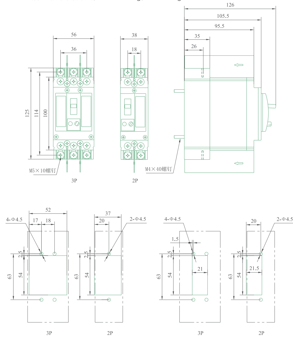
DZ931-50G 插入式安装板前接线, 重量3P约1kg, 2P约0.8kg
