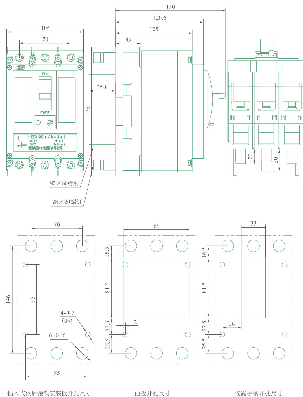
DZ931-250B/G 插入式安装板后接线，重量约3.5kg
