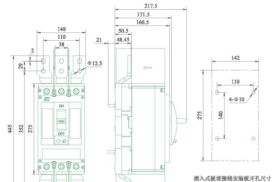
DZ931-630 插入式安装板前接线，重量约12kg
