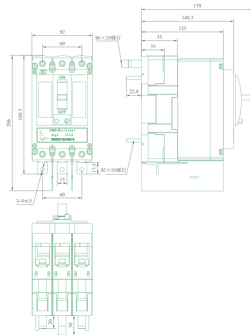
DZ931-125B/G 插入式安装电源侧板后负载侧板前接线(带电量附件或通信模块)(3P), 重量约3.4kg
